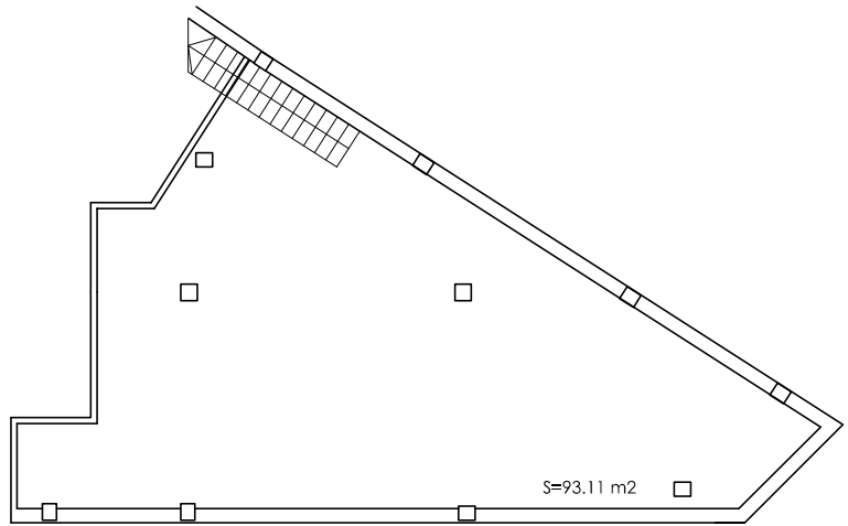
PLANTA SOTANO
